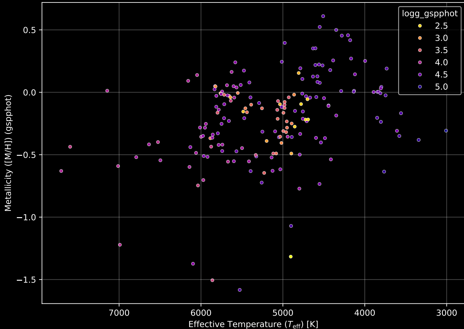
APOGEE DR17 Field: [172+58_btx] Stellar Population Parameters (n= 182)
